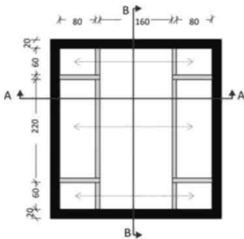
Figura 2.11 T3–Planimetri
