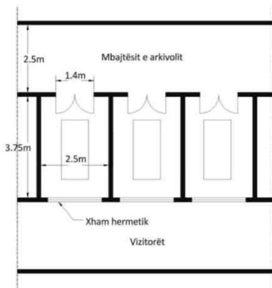
Figura 1.5 Tipologji e projektimit të morgut civil.
