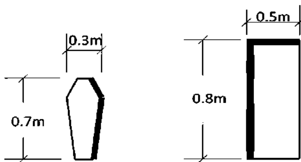
Figura 2.2 Dimensionimi i arkivolit dhe gropës së varrit për kufomat deri 1 vjeç
