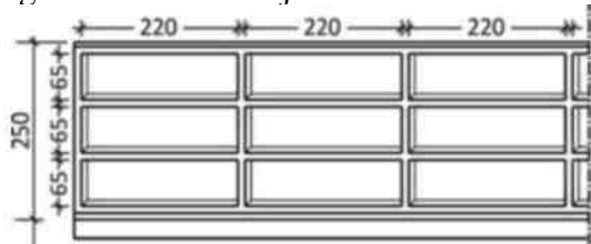
Figura 2.27 T2 – Pamje ballore
