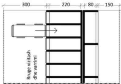
Figura 2.30 T4 – Planimetri
