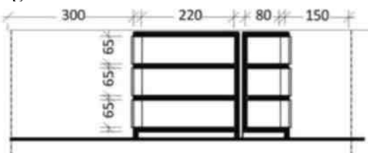
Figura 2.30 T4 – Planimetri
