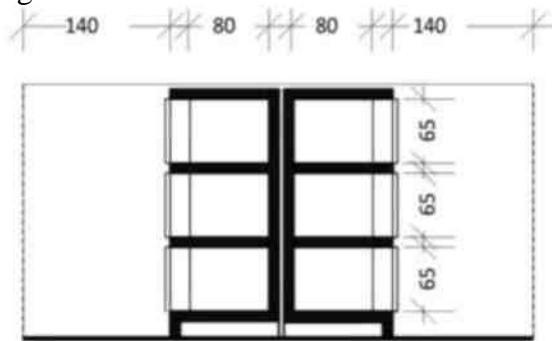
Figura 2.26 T2 – Prerje tërthore
