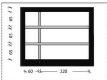
Figura 2.8 T 2 – Planimetri
