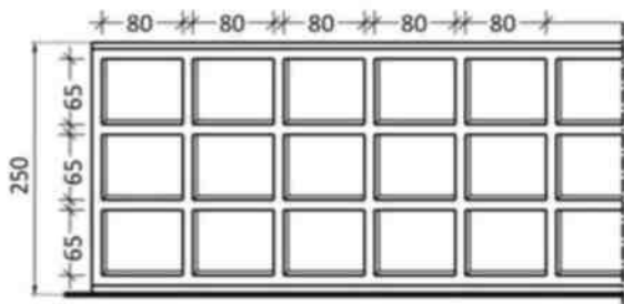
Figura 2.24 T1 –Pamje ballore
